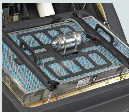
Il sistema scuoti filtro brevettato (a frequenza armonica variabile) garantisce l'ottimale pulitura del filtro in tutte le sue parti
